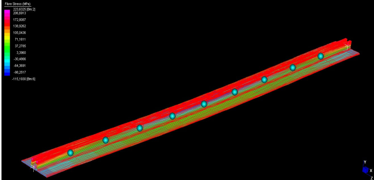
Diagramma delle tensioni. Diagramma di carico a rottura
